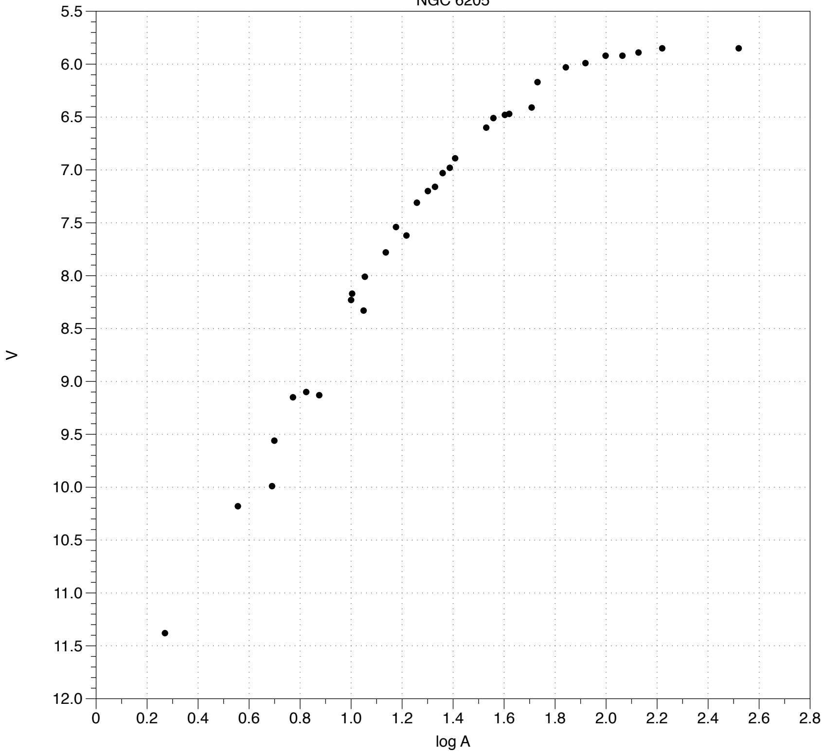
NGC 6205
